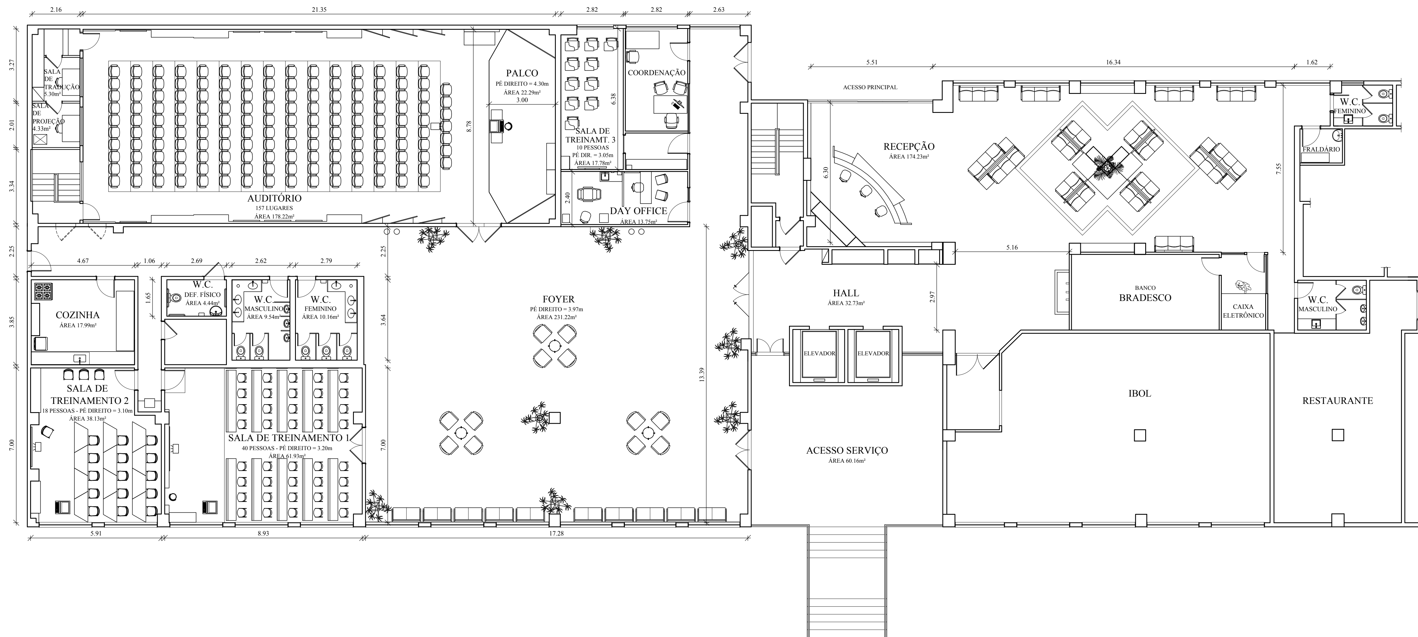
PLANTA BAIXA DO PRIMEIRO ANDAR – BLOCO 2
